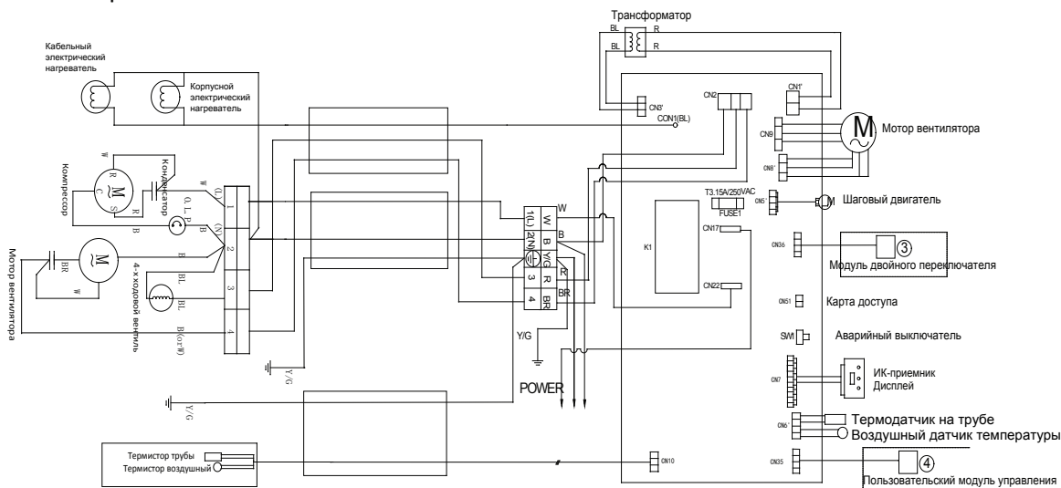
Эл.Схема Внешнего блока
